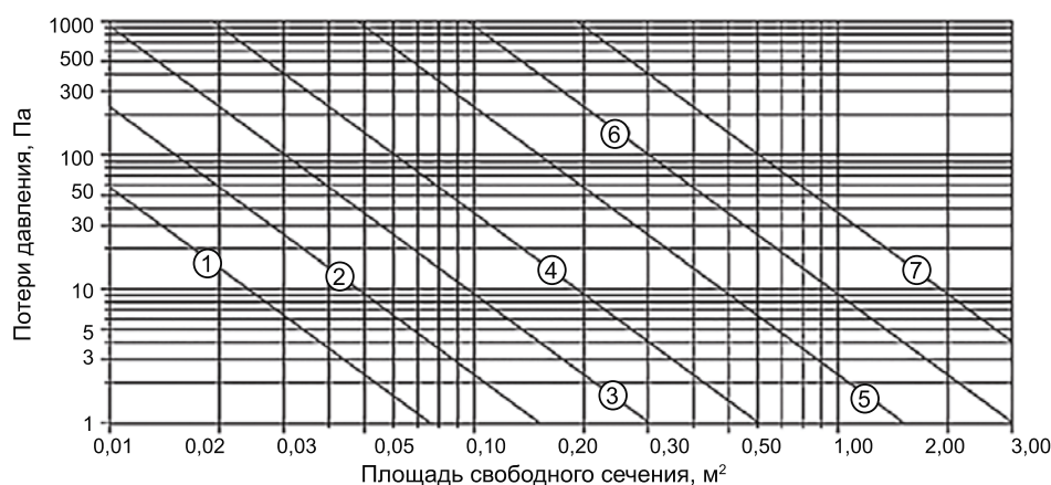
Диаграмма зависимости потери давления от площади свободного сечения решеток РВНС, РВННС
