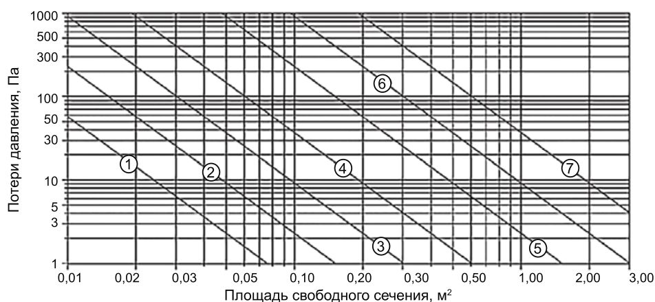
Диаграмма зависимости потери давления от площади свободного сечения решеток РВНС, РВНС
