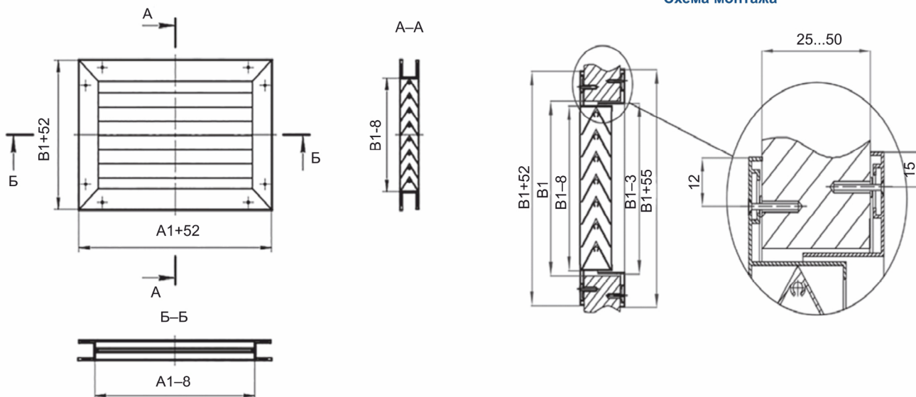
Схема монтажа
