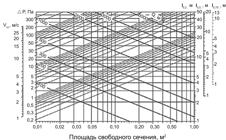
Диаграмма зависимости потери давления от площади свободного сечения решеток РВ1
