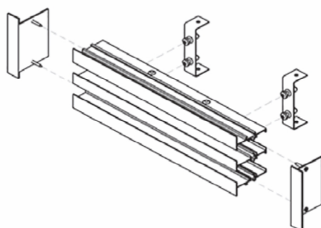
Схема монтажа решетки с дополнительными кронштейнами
